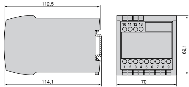
Fig. 7. Boîtier type P13/70 encliqueté sur rail «à chapeau» (35 × 15 mm ou 35 × 7,5 mm, selon EN 50 022).
